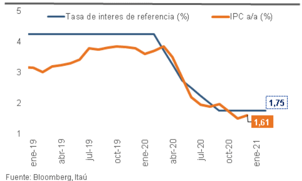
Colombia: Tasa de intervención vs Inflación anual (%)
